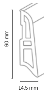
Döllken uitbrektang
