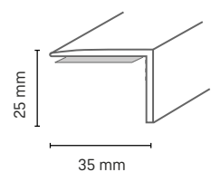
zelfklevende variant
